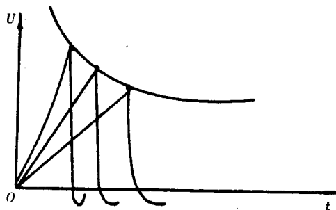
图 10 线性上升冲击伏秒特性曲线
