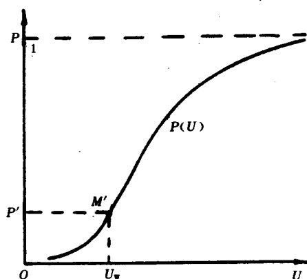
图 3 统计操作[雷电]冲击耐受电压 U_w
